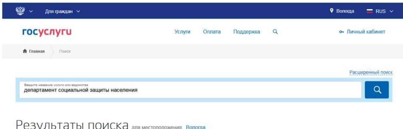
Рисунок 2. Сортировка услуг
