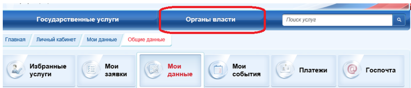
Рисунок 2. Сортировка услуг
